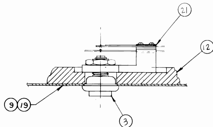
SEC A-A
