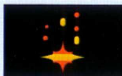
SOLAR FLARES
