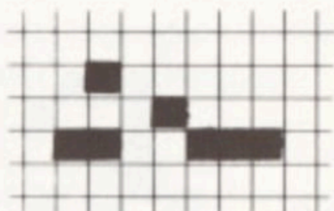
Acorn
