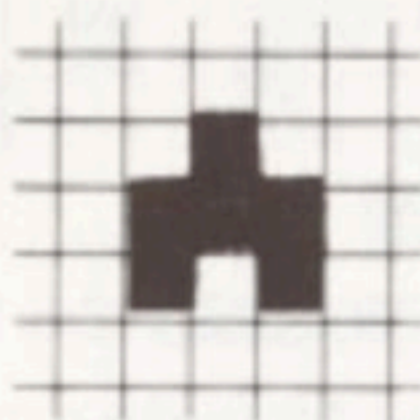
Blasting cap
