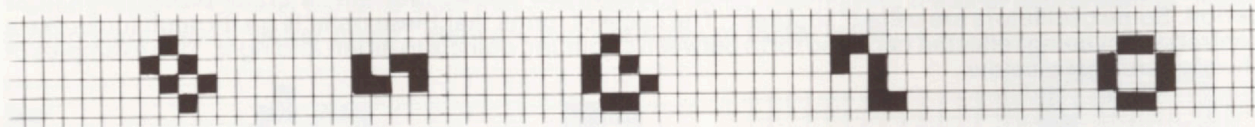
Pond
