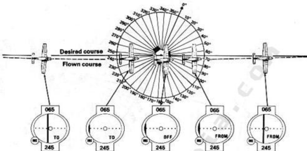
Figure 14. VOR Passage
