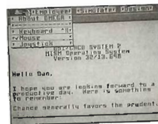
Diagram 1.1.1 --SYSTEM Menu
