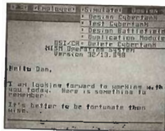
Diagram 1.1.4 --DESIGN Menu
